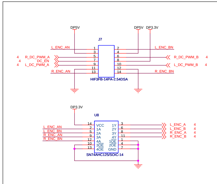
DC MOTOR
